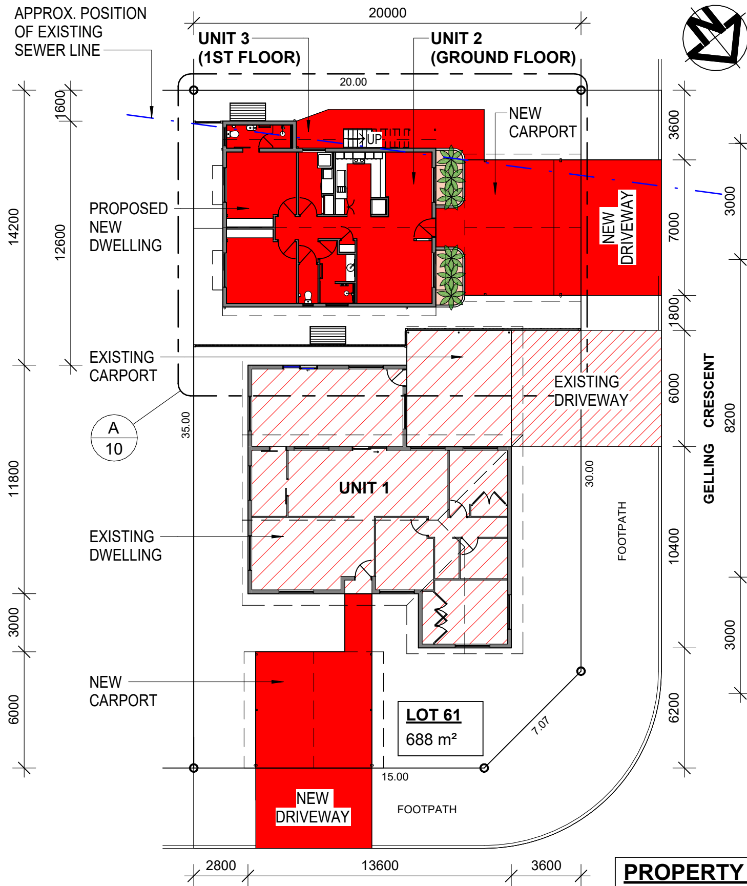
SITE LAYOUT PLAN SCALE: 1 : 200
