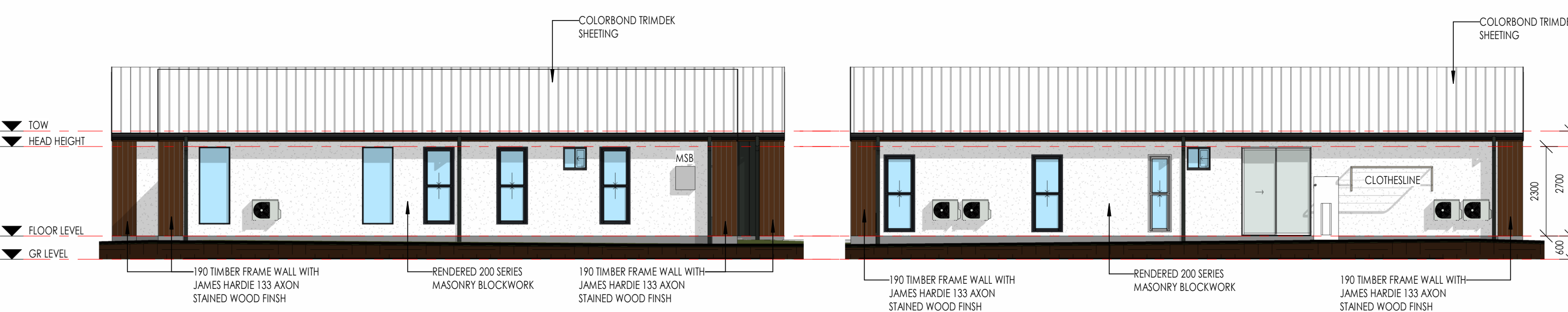
ELEVATION 2 1 : 100
