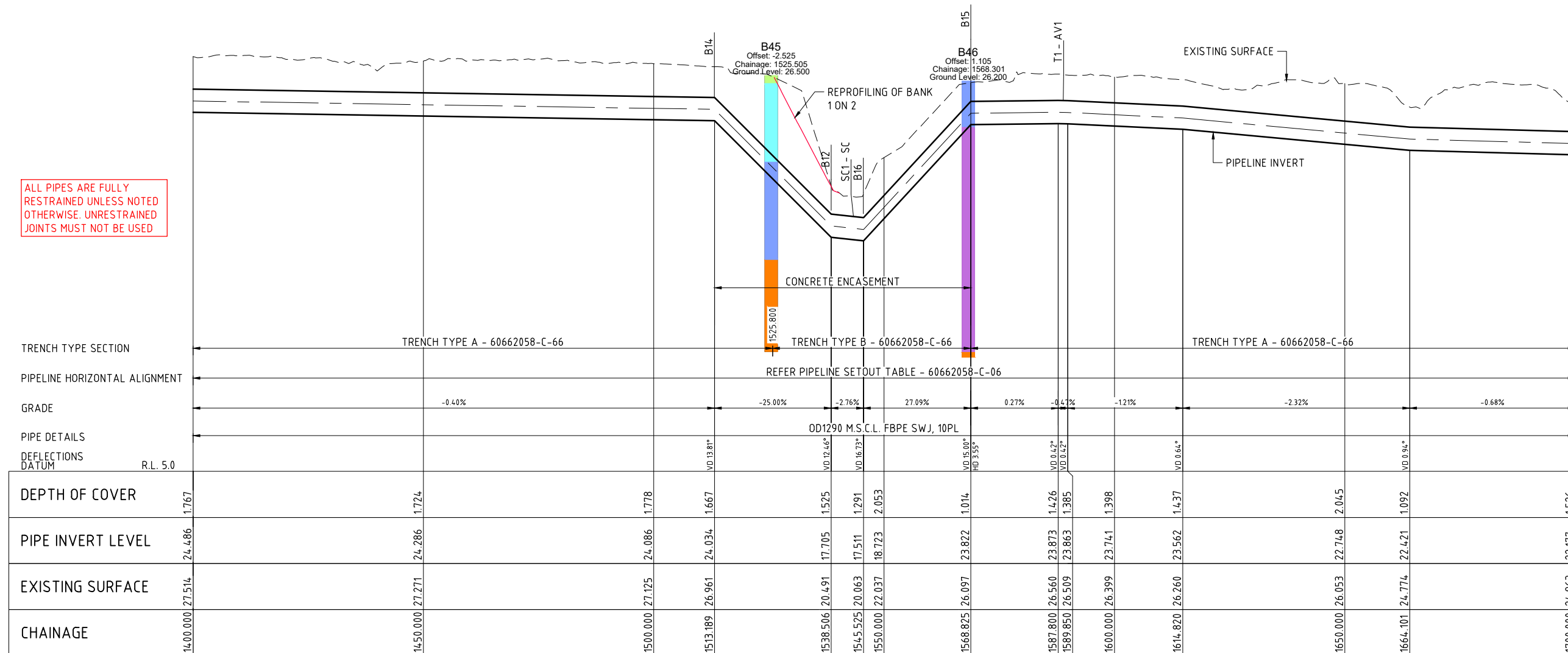
LONGITUDINAL SECTION
