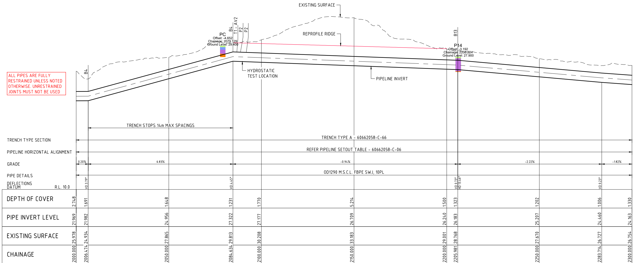
LONGITUDINAL SECTION
