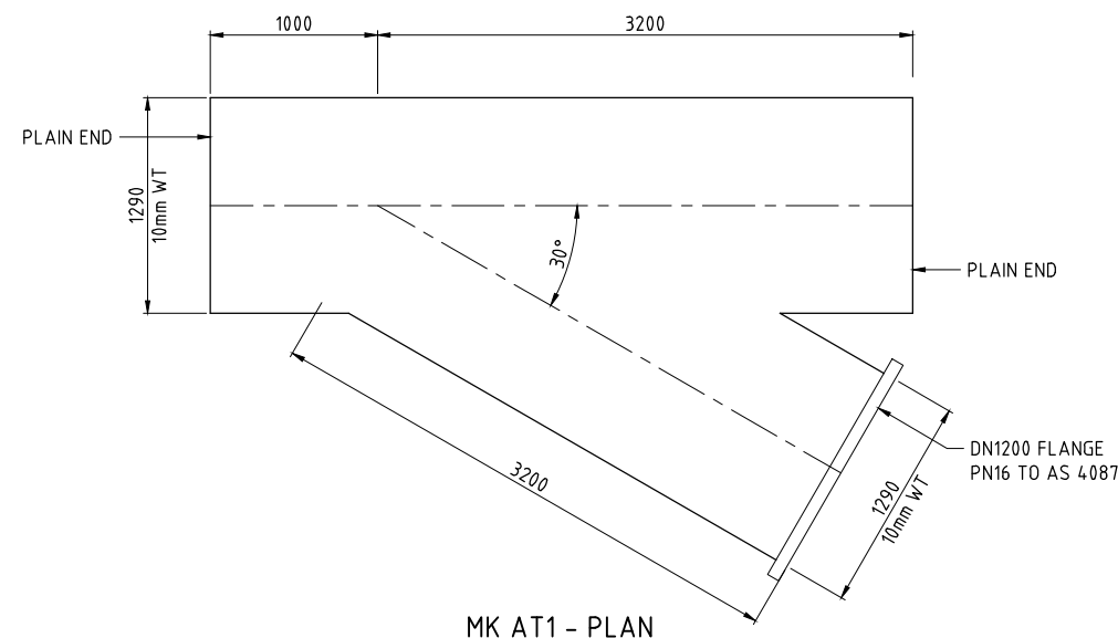
MK AT1 - PLAN
