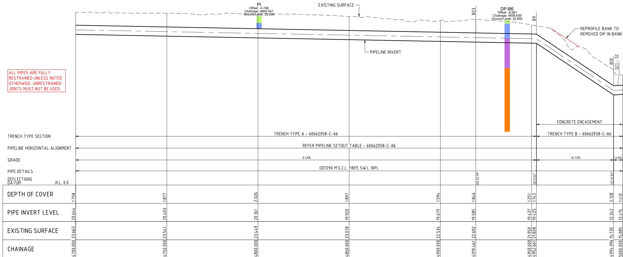
LONGITUDINAL SECTION
