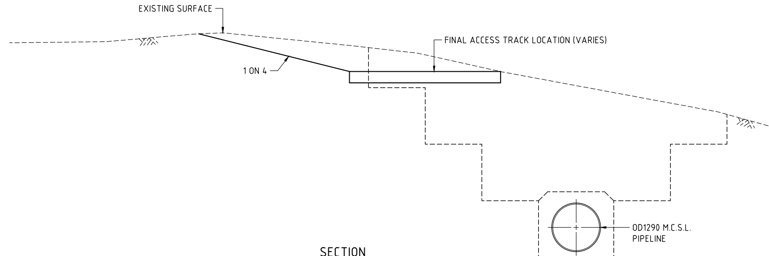
SECTION CH 7560
