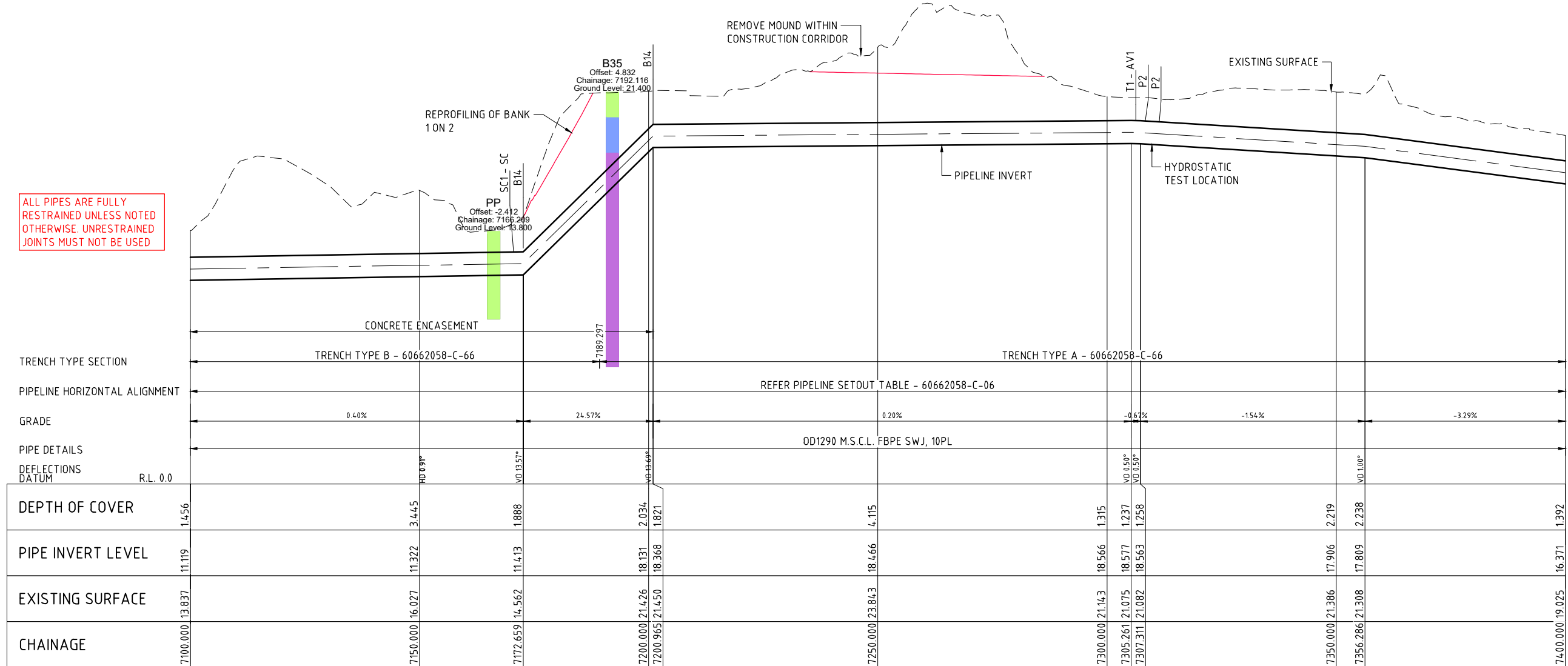
LONGITUDINAL SECTION
