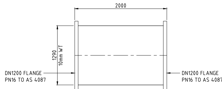
MK P6 - PLAN
