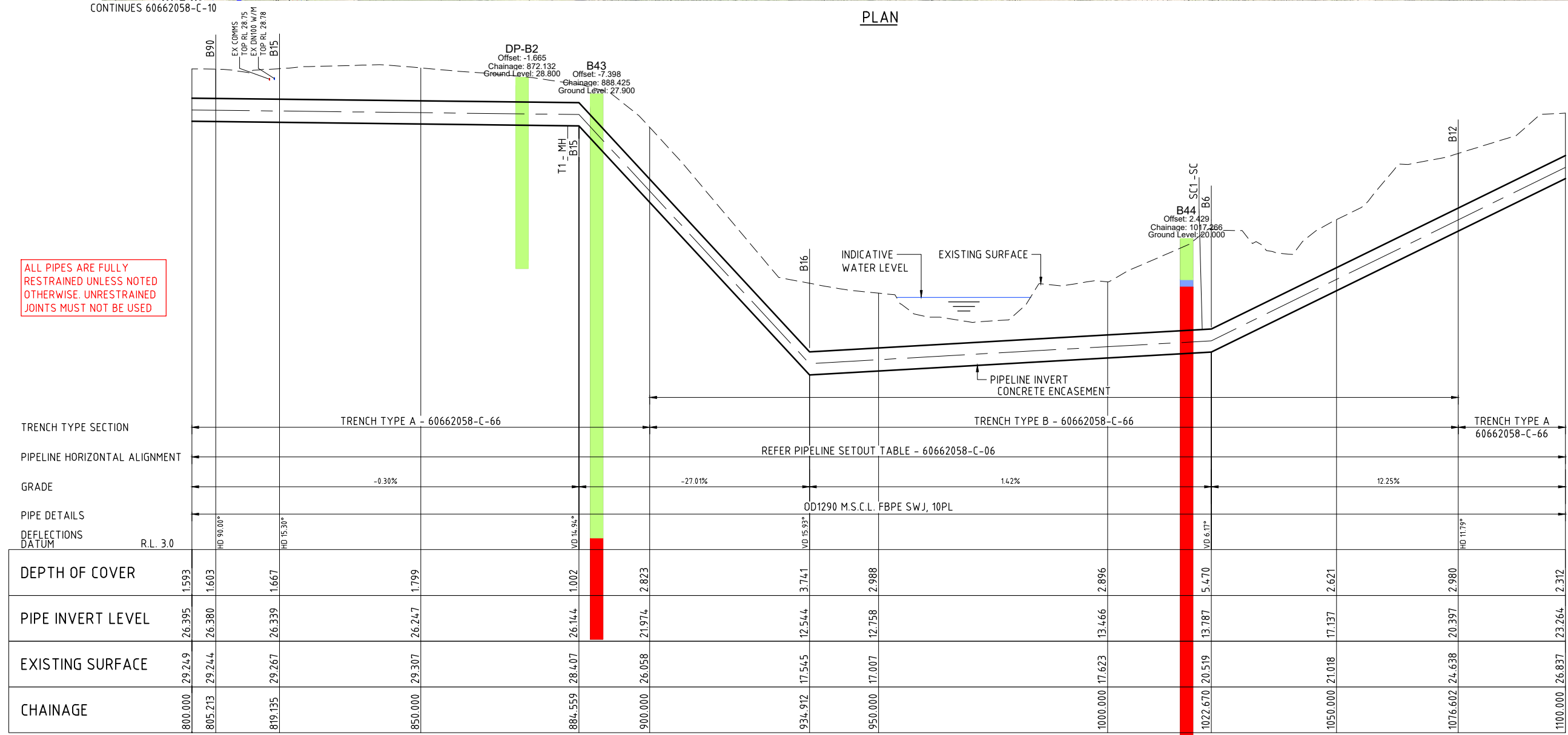
LONGITUDINAL SECTION
