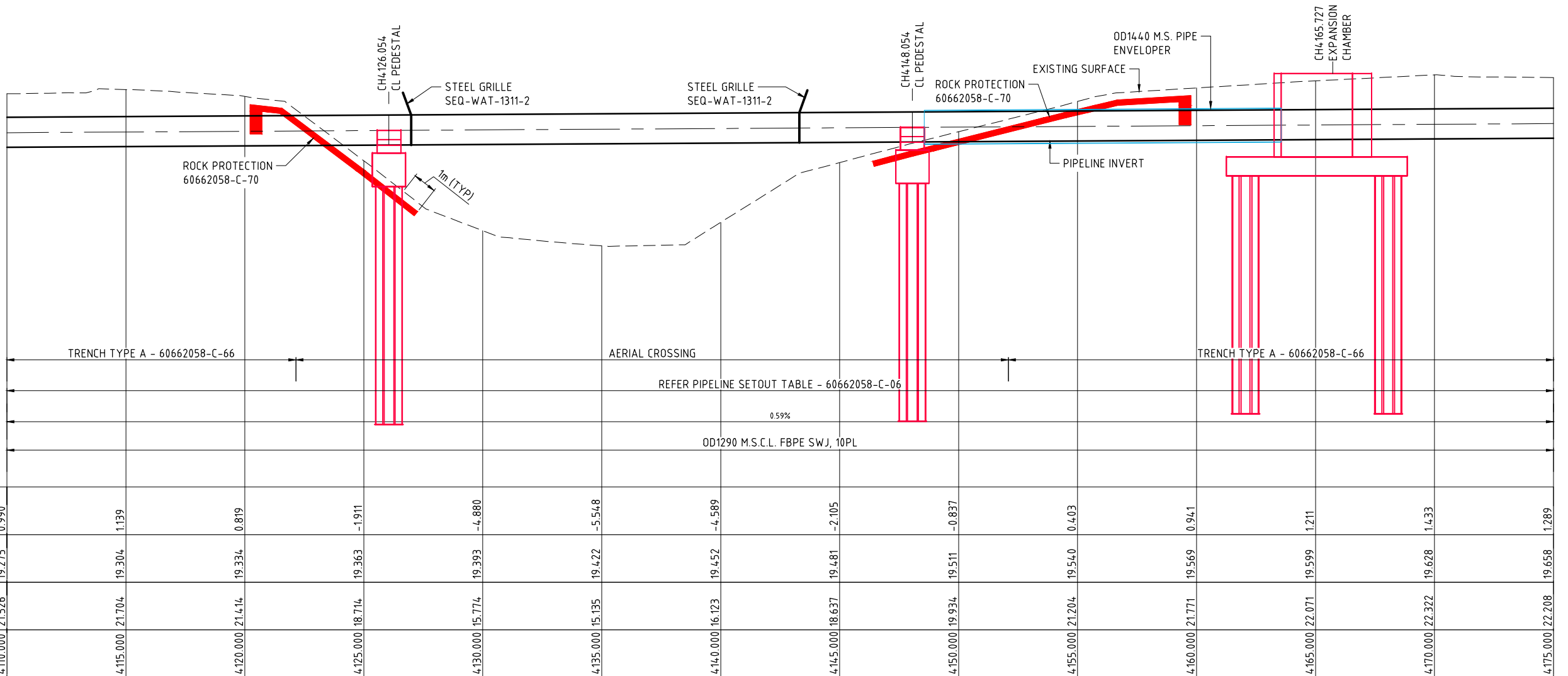
LONGITUDINAL SECTION
