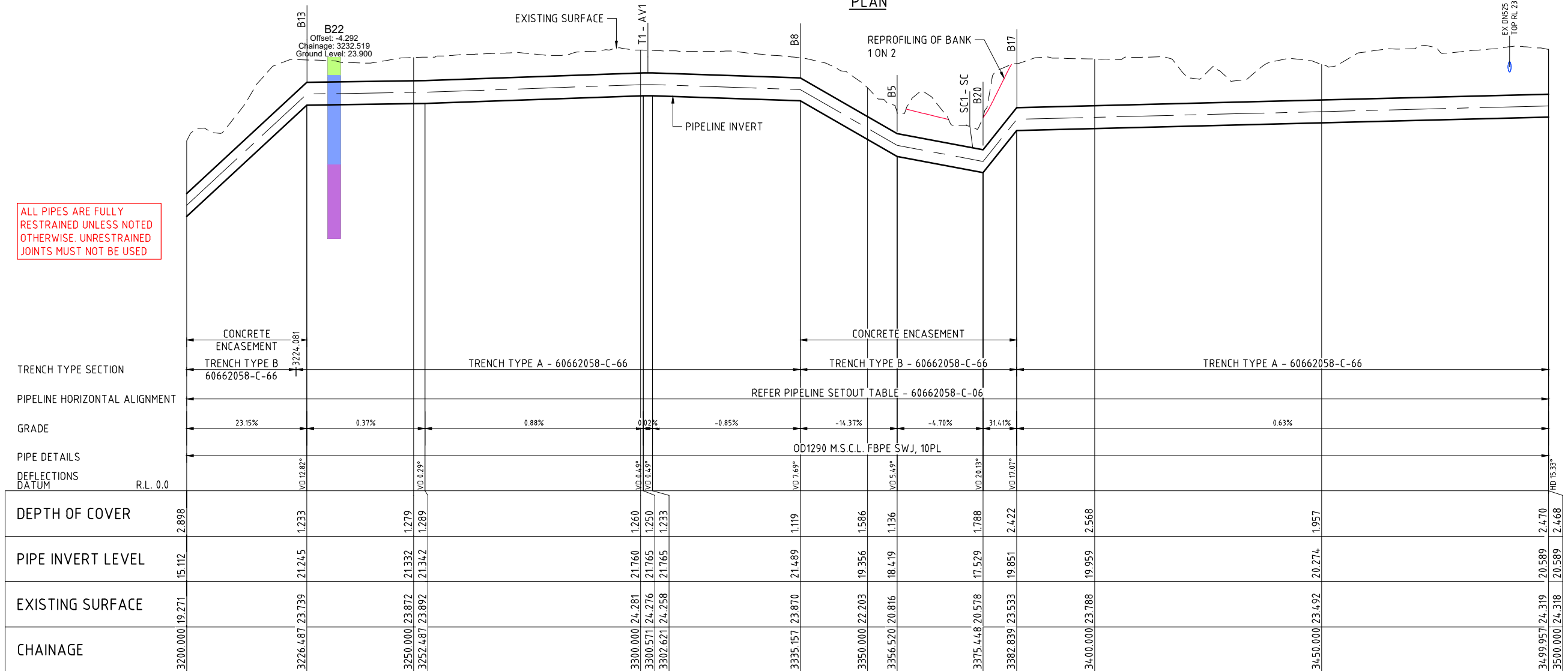
LONGITUDINAL SECTION
