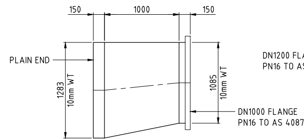
MK RE4 - ELEVATION
