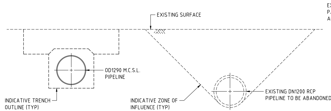
SECTION CH 100
