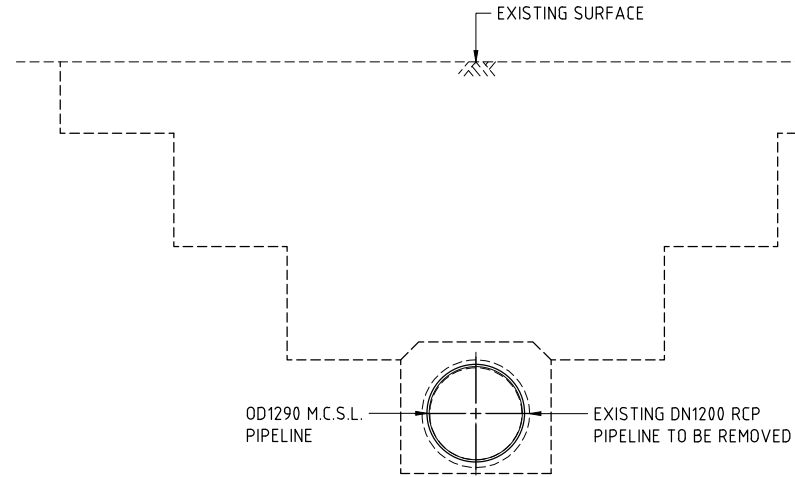
SECTION CH 525
