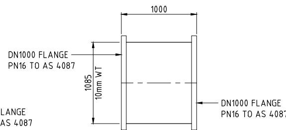
MK P3 - PLAN
