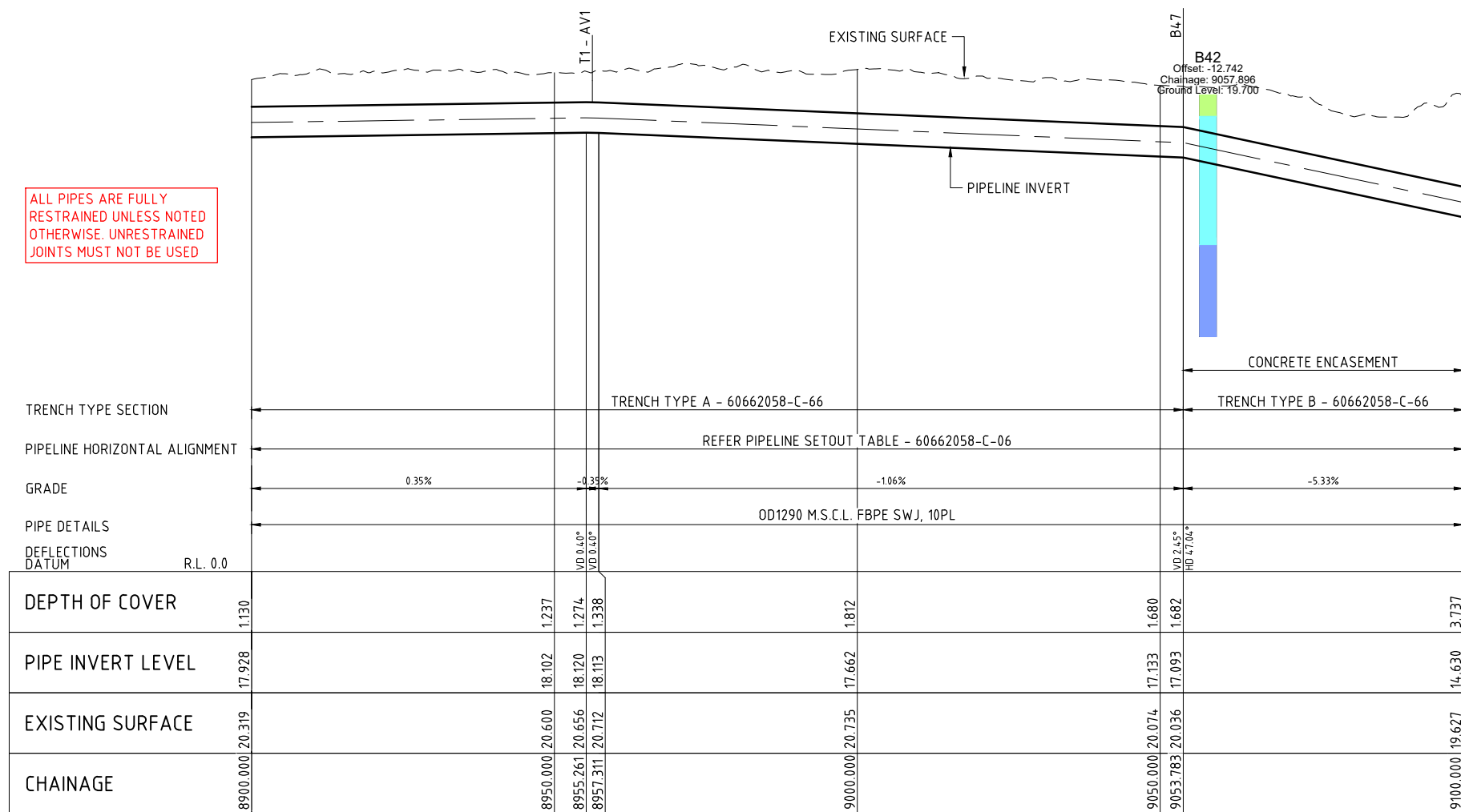
LONGITUDINAL SECTION
