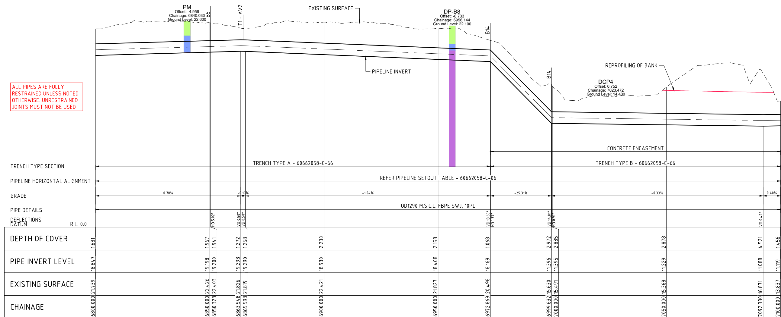
LONGITUDINAL SECTION
