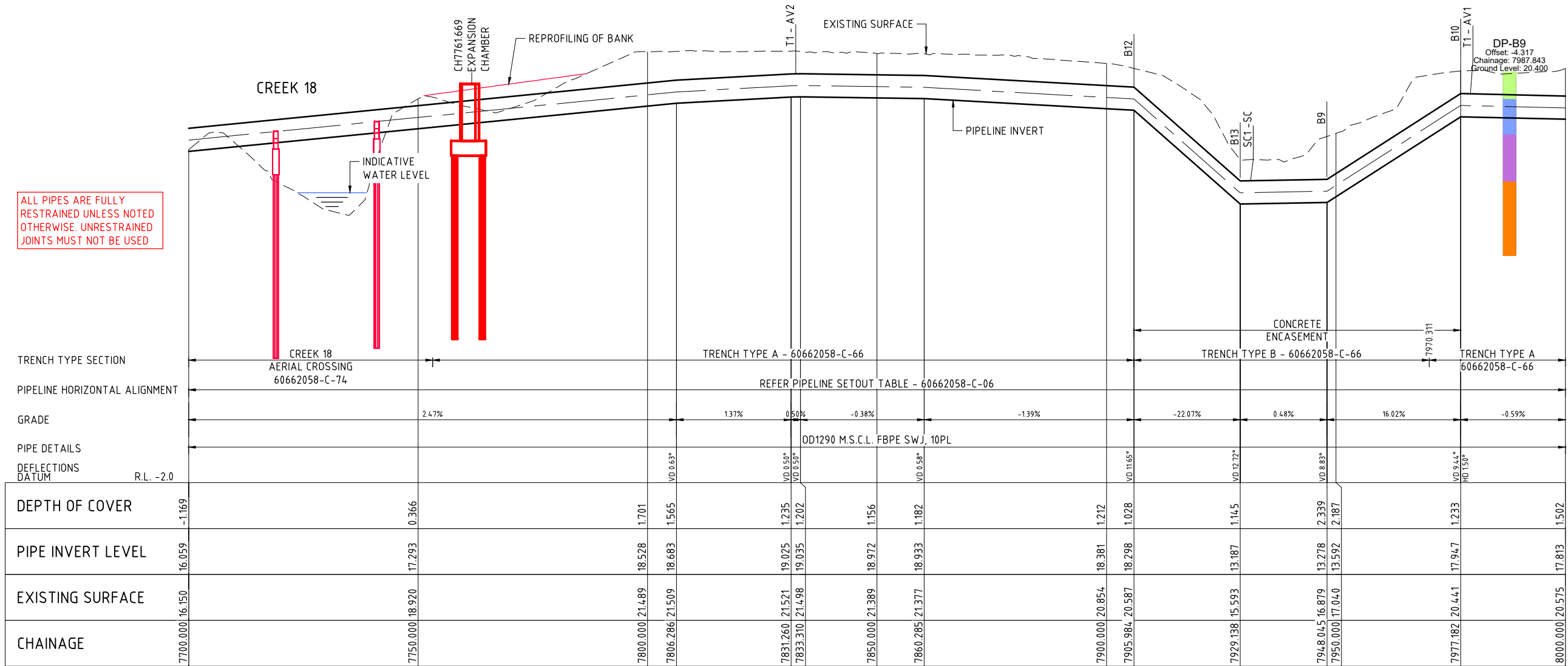
LONGITUDINAL SECTION
