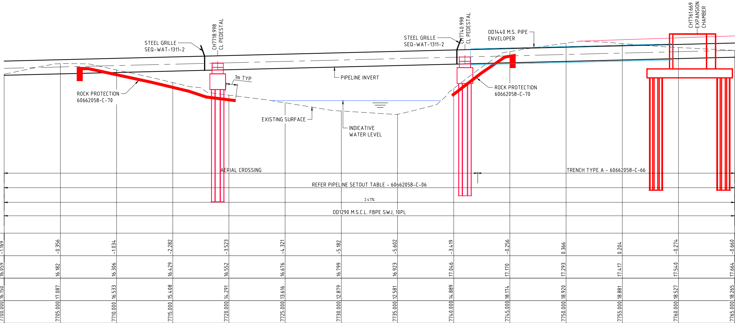
LONGITUDINAL SECTION
