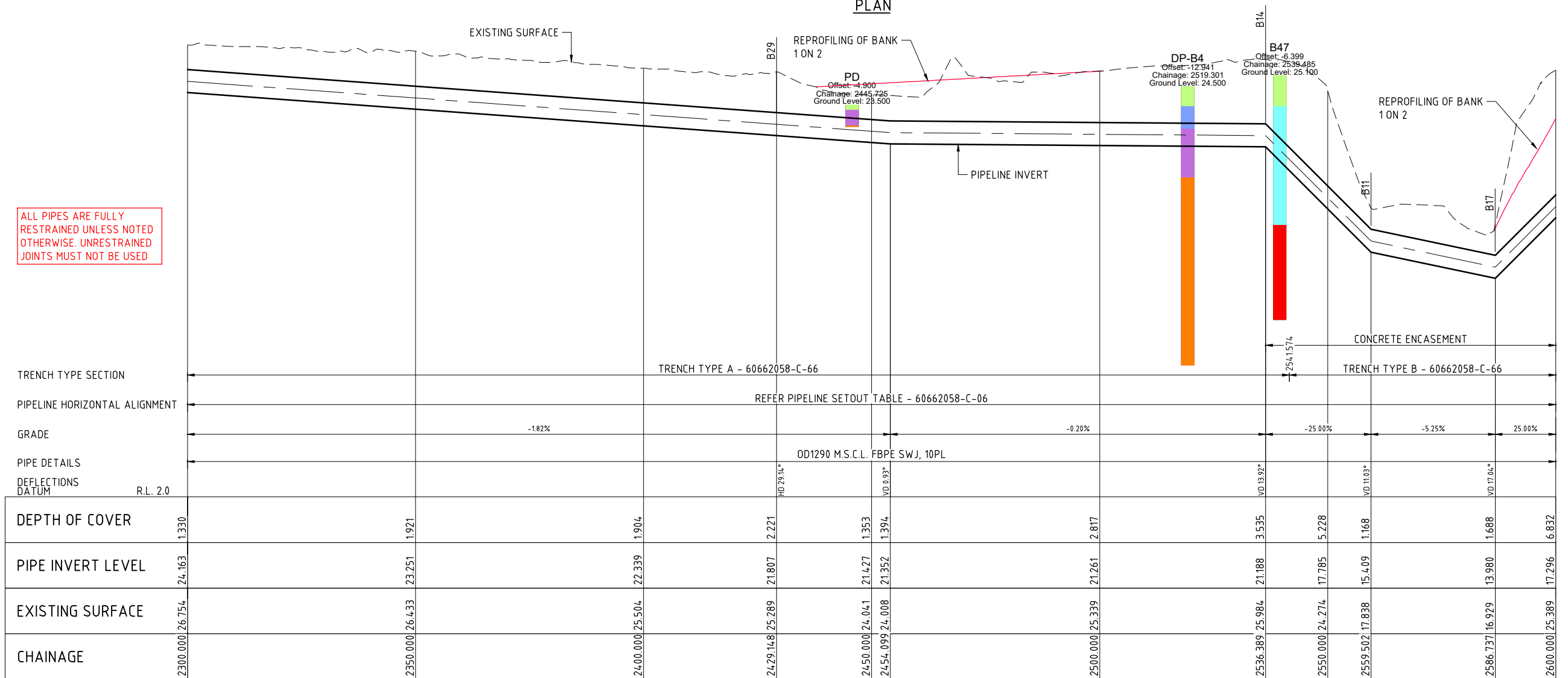
LONGITUDINAL SECTION
