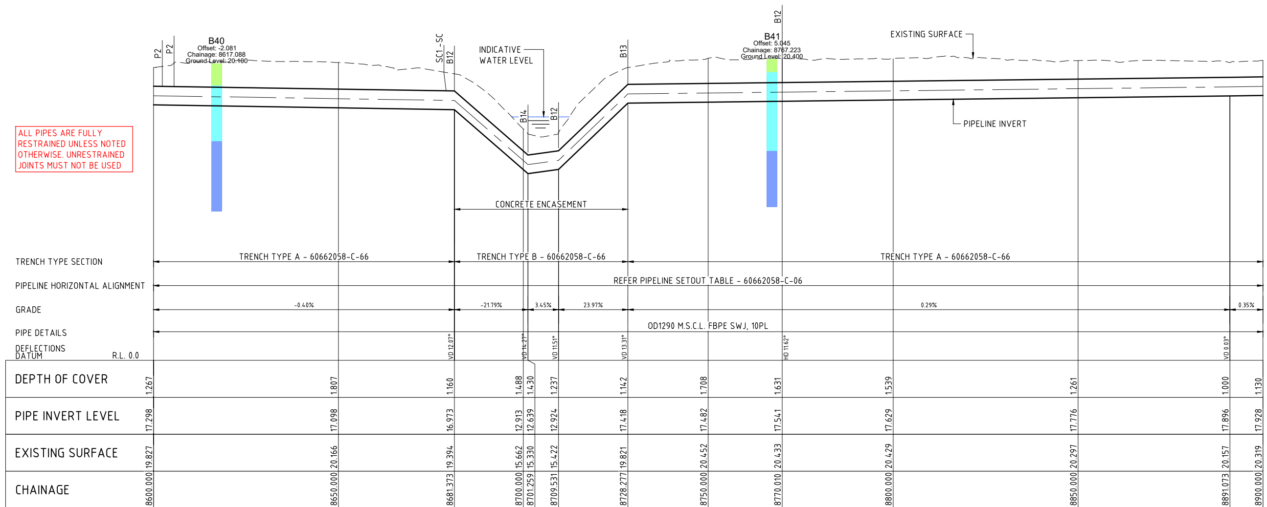
LONGITUDINAL SECTION
