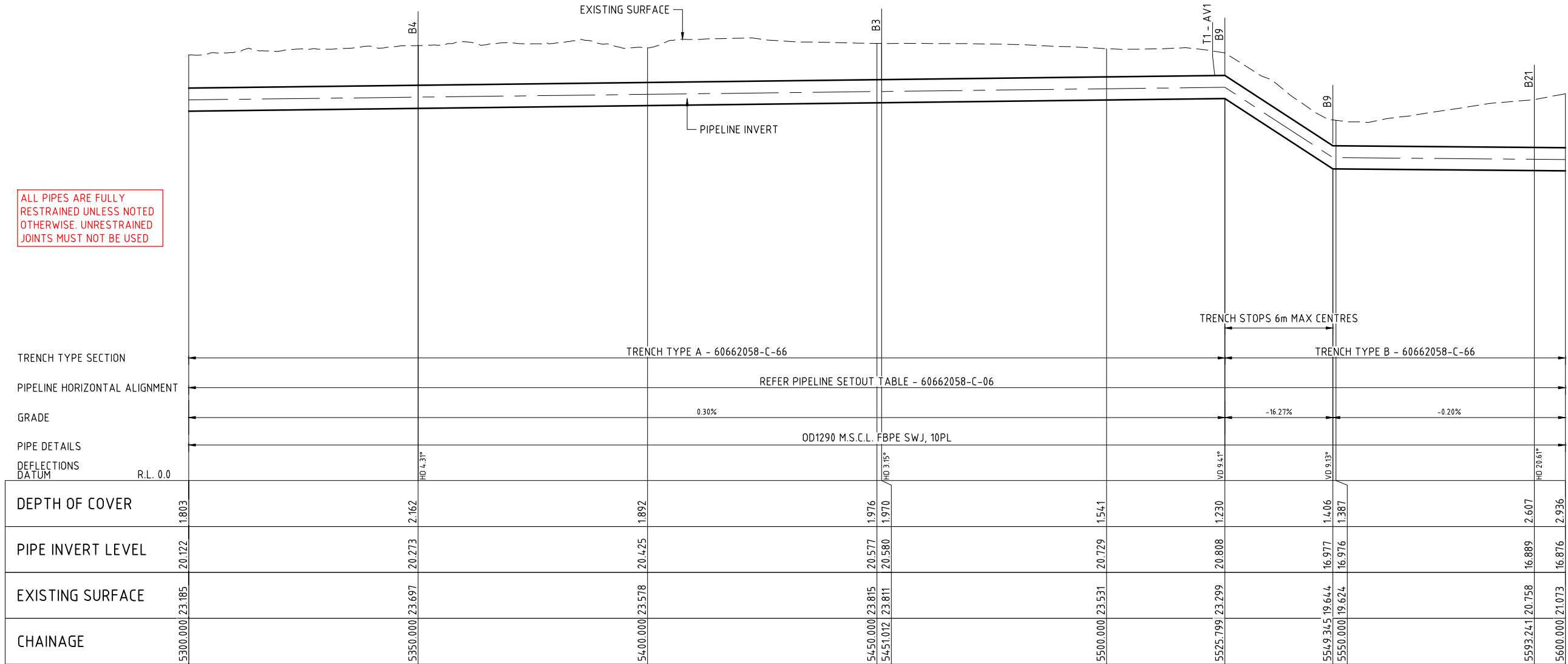
LONGITUDINAL SECTION
