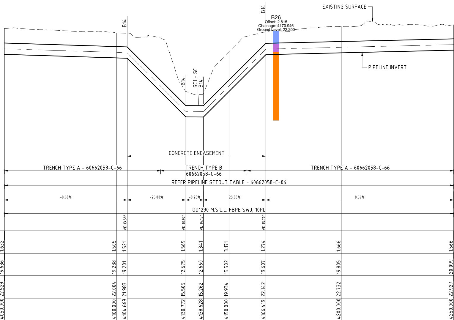
LONGITUDINAL SECTION
