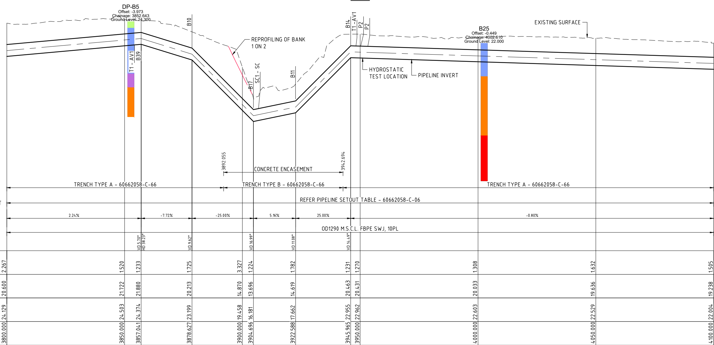
LONGITUDINAL SECTION
