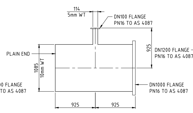
MK T4 - ELEVATION
