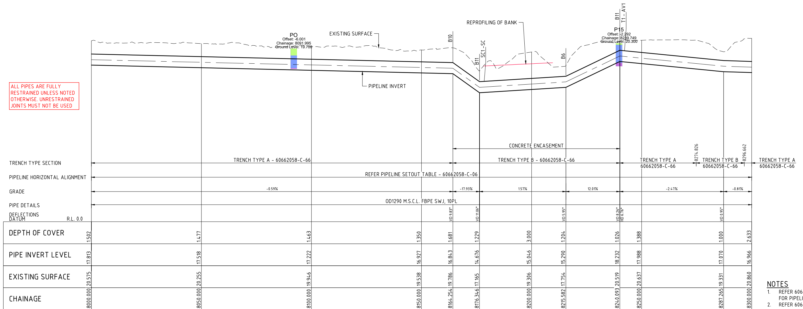
LONGITUDINAL SECTION
