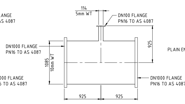
MK T3 - ELEVATION
