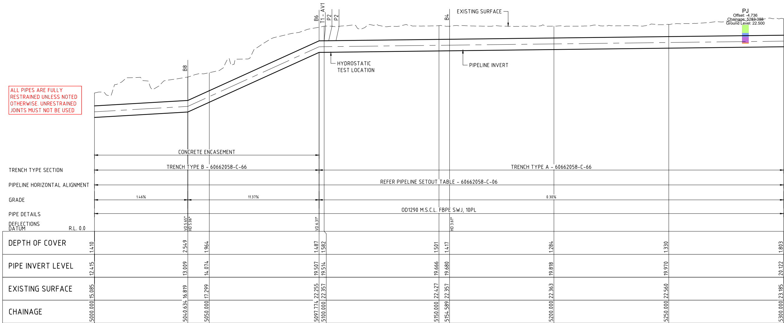
LONGITUDINAL SECTION
