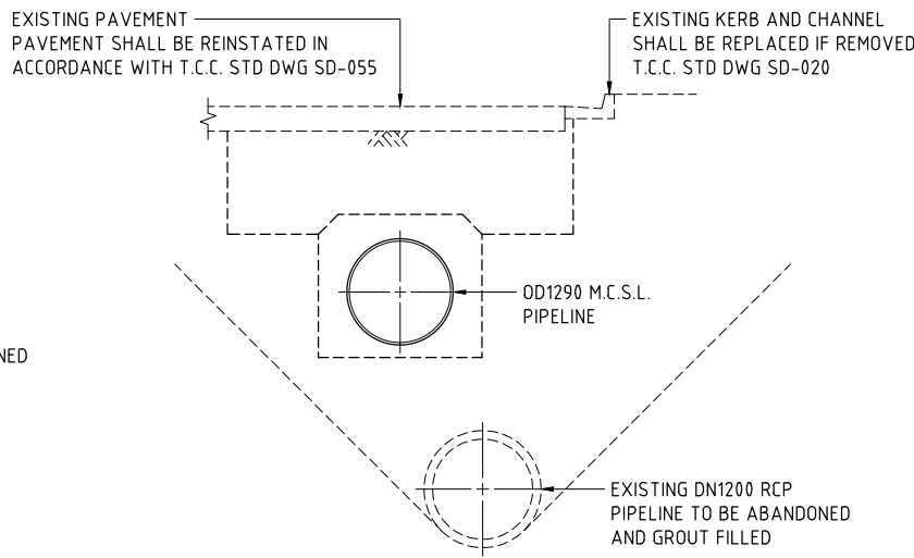
SECTION CH 400
