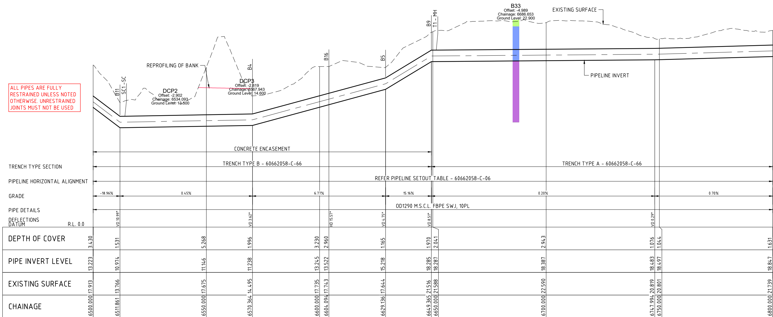
LONGITUDINAL SECTION
