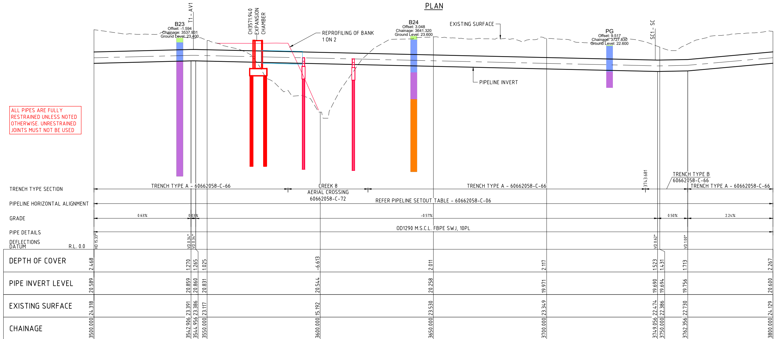
LONGITUDINAL SECTION
