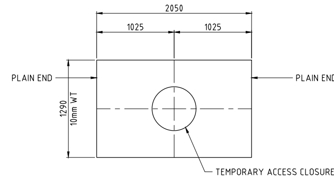
MK P4 - PLAN
