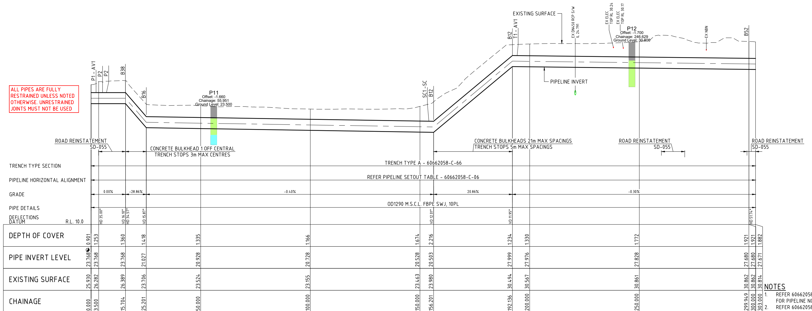
LONGITUDINAL SECTION
