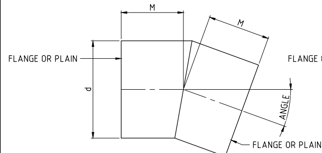
MK B(ANGLE) 0° TO 22.5° MITRED BEND
