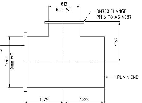
MK T6 - ELEVATION
