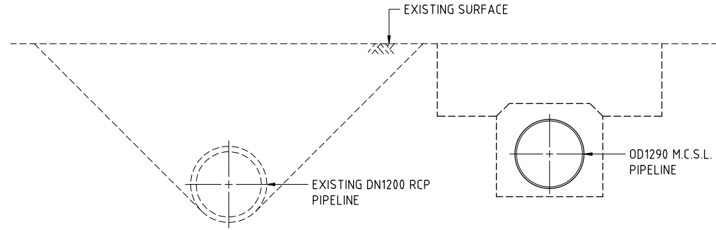
SECTION CH 9200
