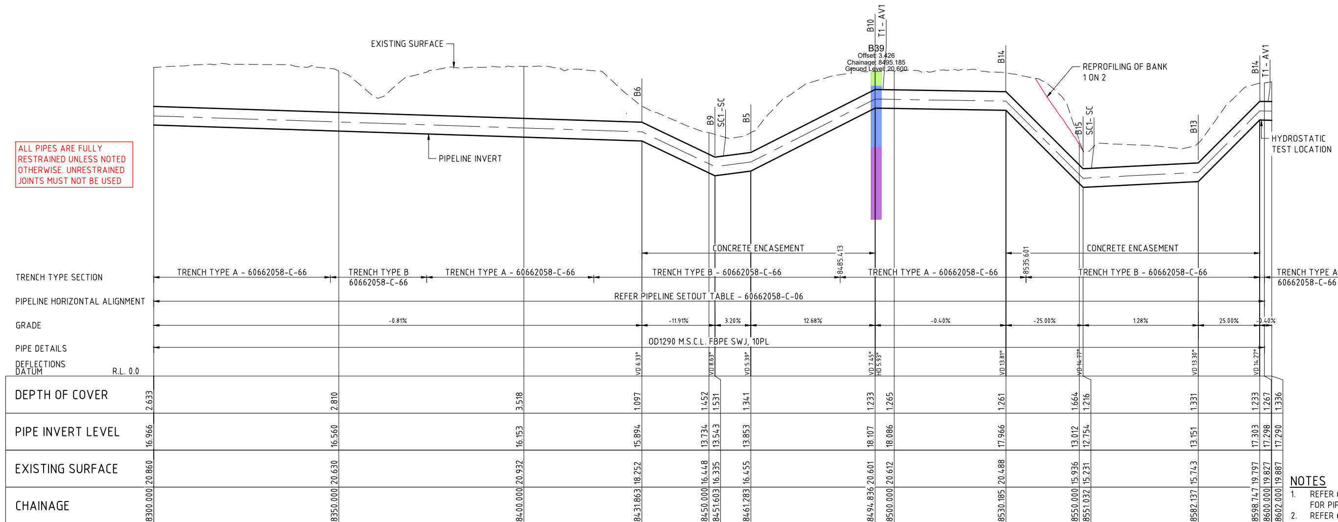
LONGITUDINAL SECTION
