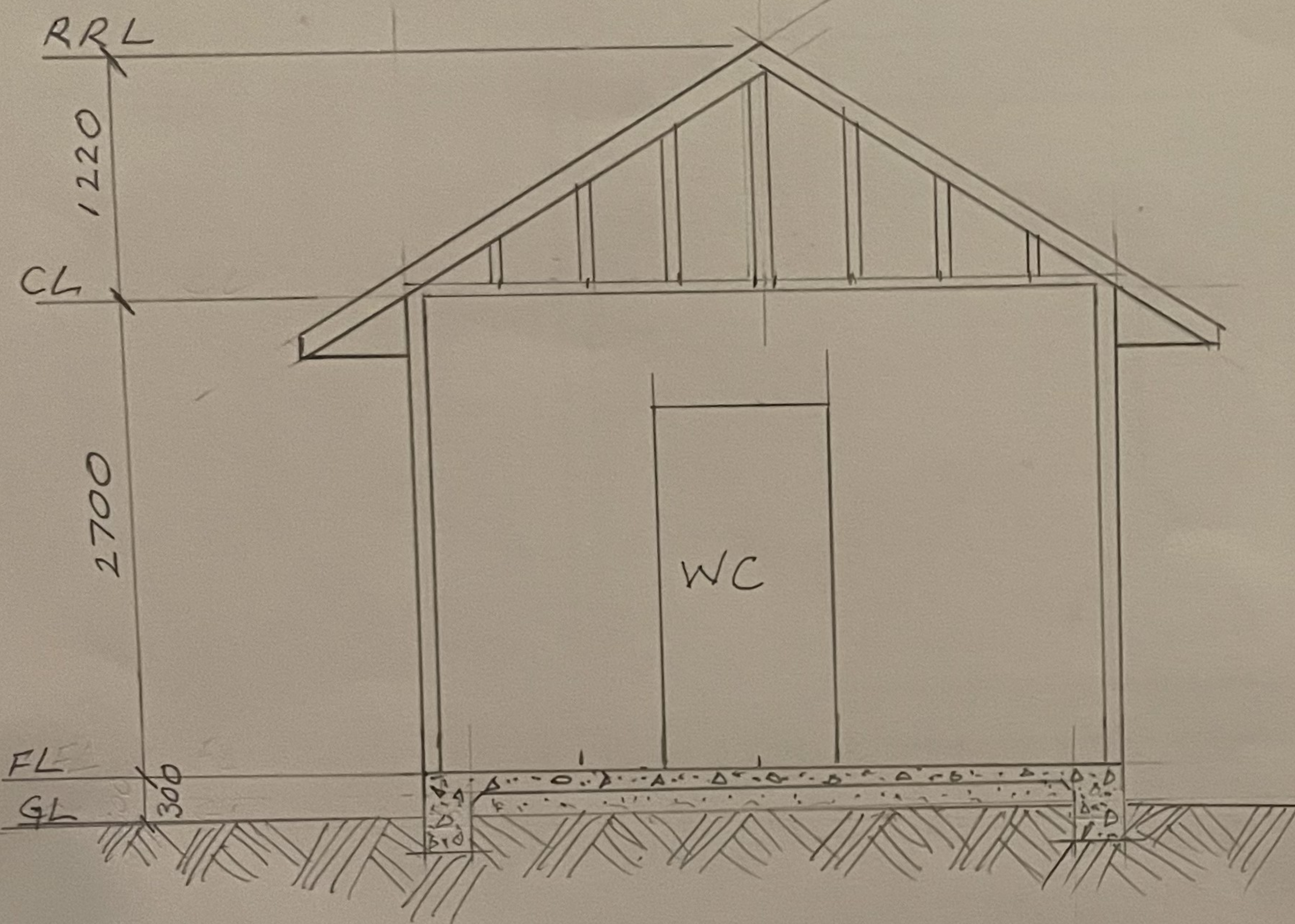
SECTION A-A 1:50
