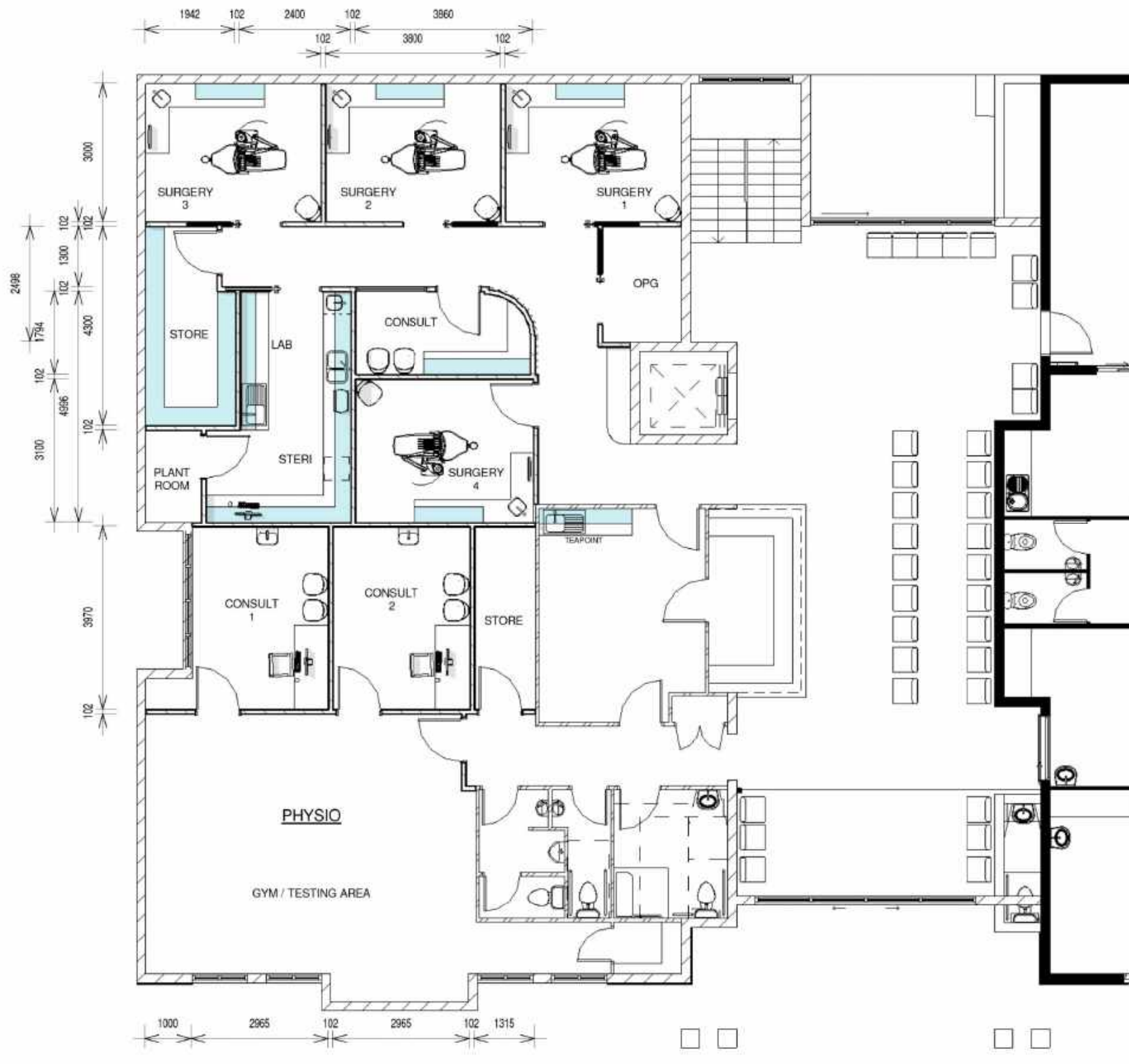
1 Upper Floor Plan 1 : 100
