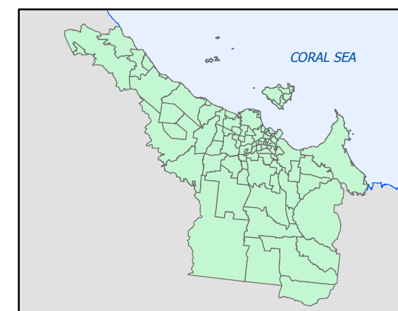
Overlay Map - OM-08
